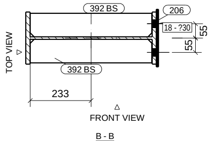
B - B
